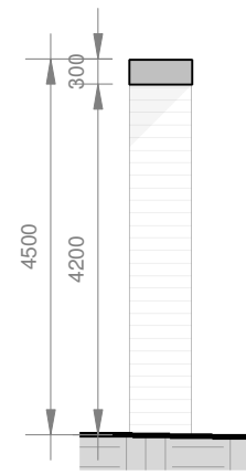
Section B-B 1 : 100
