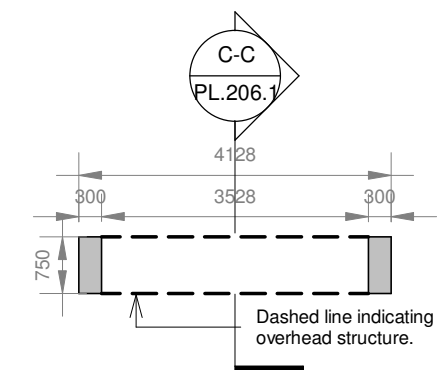
Corten Steel Portal - 03 1 : 100
