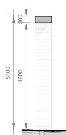
Section C-C 1 : 100
