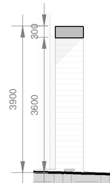
Section A-A 1 : 100
